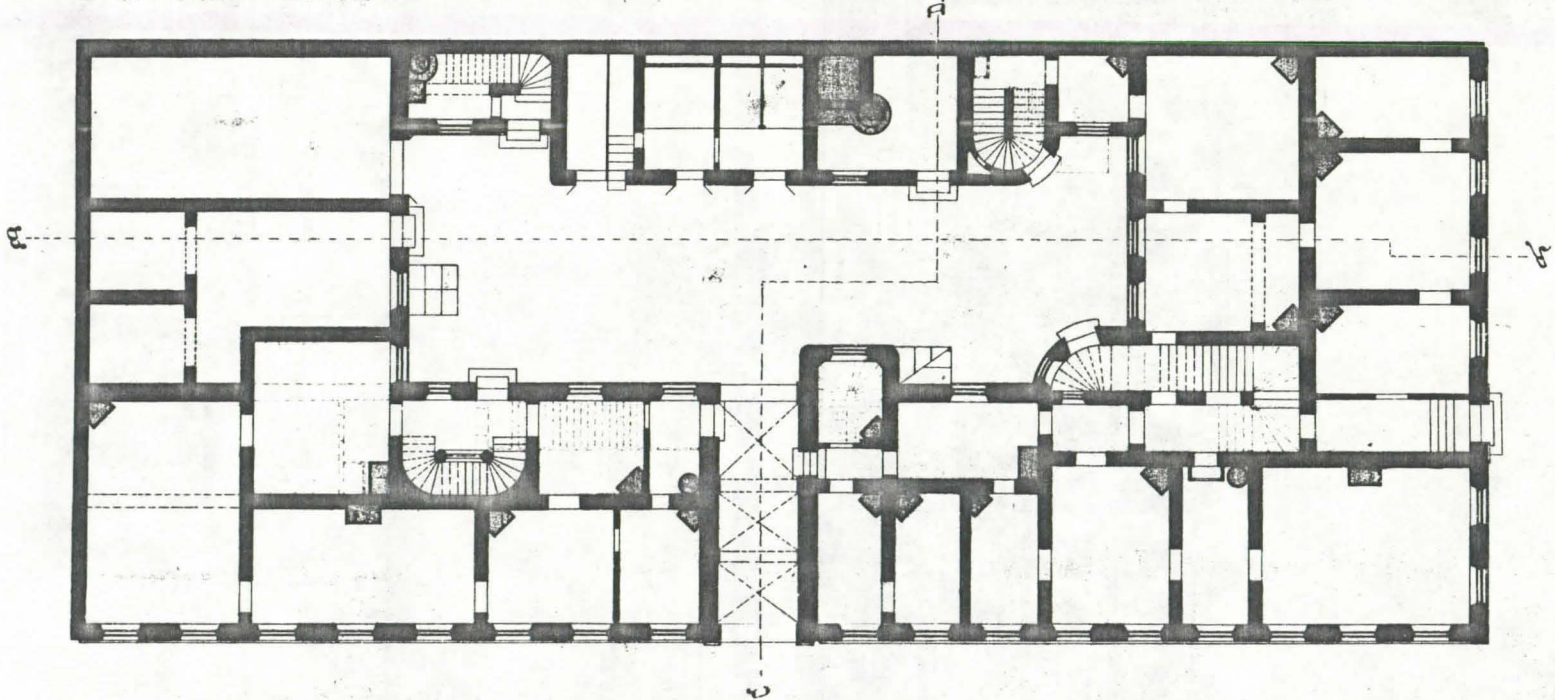
PLAN AF BOTTENVÄNGEN.
