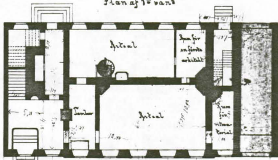
Plan af 1 te vån.
