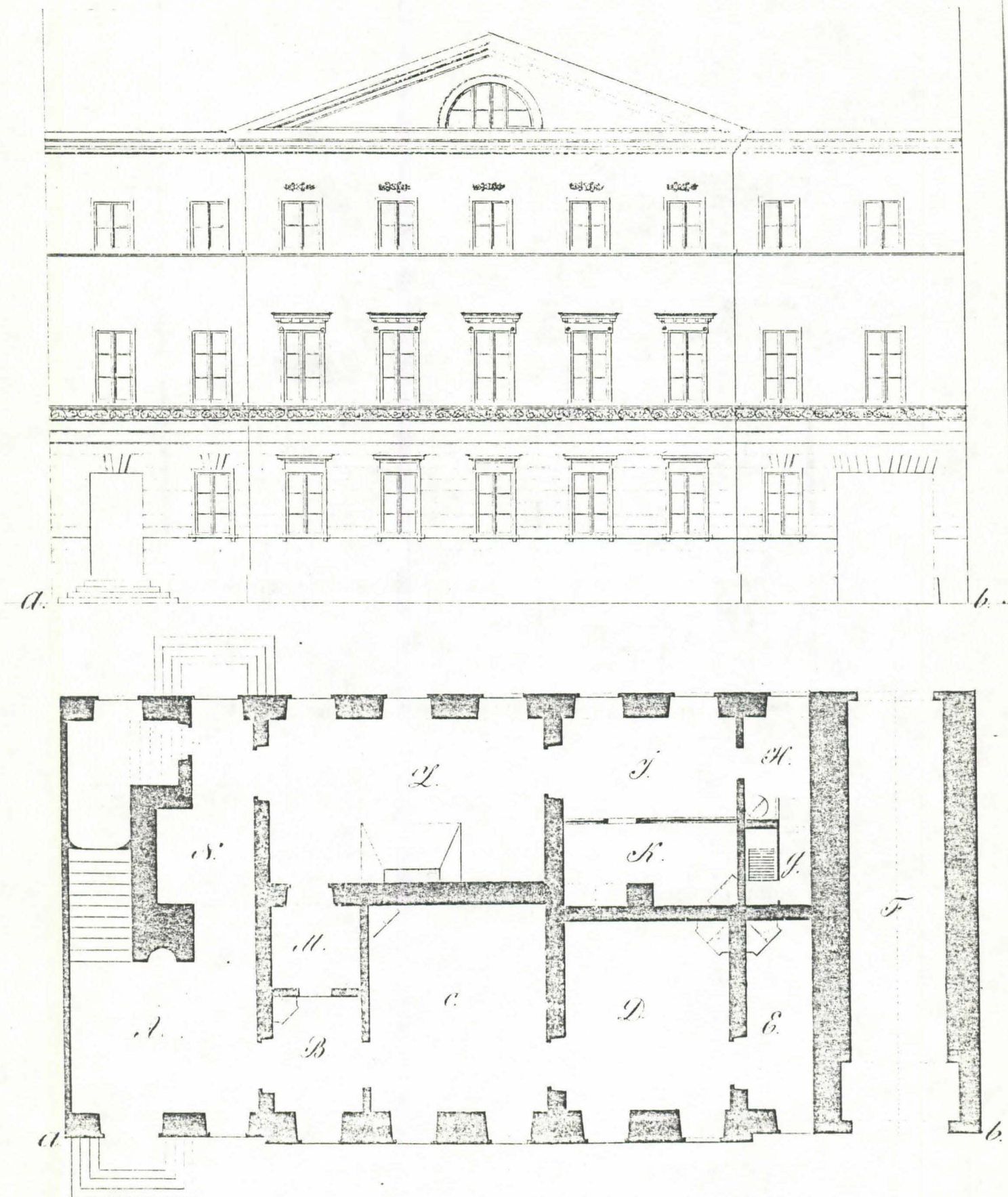
Kuva 2. Salaneuvos Walleenin talo. Aleksanterinkatu 8, julkisivu ja ensimmäinen kerros. Urakkatajouskilpailun asiakirjojen liitepiirustukset 1853. VA. Senaatin talousosasto.
