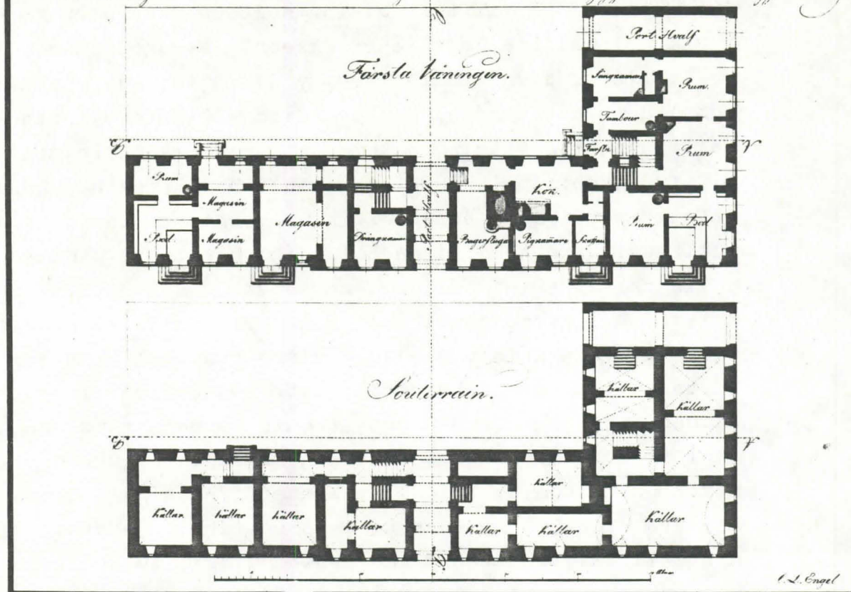
Kuvat 1 ja 2. Carl Ludvig Engelin suunnitelma raatimies Erik Borgströmin taloksi Mariankadun ja Aleksanterinkadun kulmantontille. Kellari- ja asuinkerrosten pohjat. VA. RHA.
