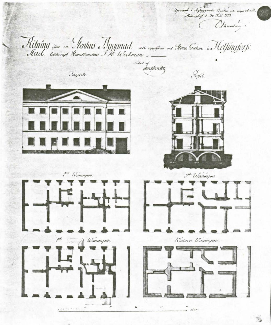
Kuva 1. Anders Kocken suunnitelma kauppias Weckmanin kivitaloksi 1813. Huomiota kiinnittää ikkunakorkeuksien erilaisuus. Vastaavanlainen ikkunajäsentely oli myös naapuritalossa eli Sederholmin talossa, ks. Aleksanterinkatu 6, liite 1 s. 5,6. VA. RHA.
