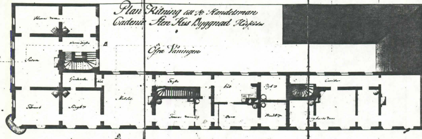
Kuvat 1 ja 2. Pehr Granstedtin suunnitelma kauppias Cadeniuksen taloksi 1817. Kaksikerroksisen kulmatalon pääjulkisivu oli Aleksanterinkadulle (silloiselle Suurkadulle). Neliömäisessä julkisivussa on vielä hyvin kustavilainen yleisleima. VA. RHA.
