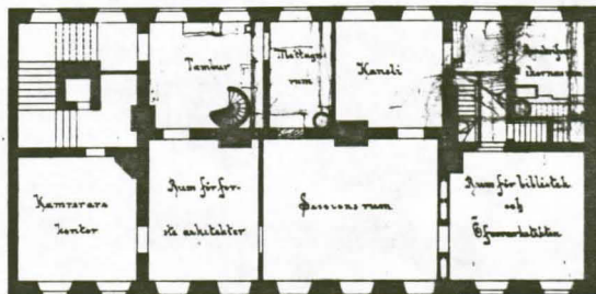
Plan af 4 te vån.
