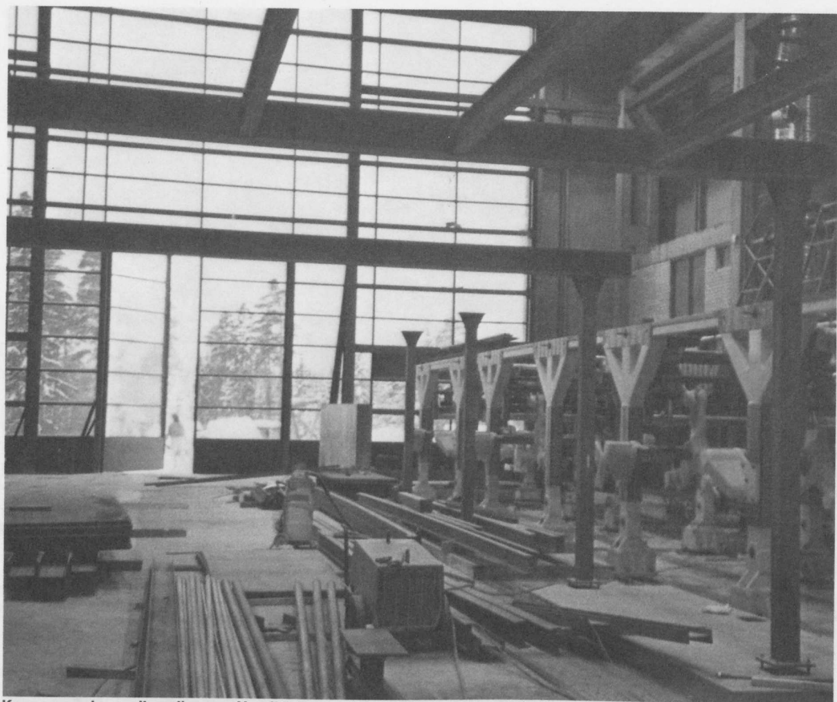
Koneasennuksen alkuvaiheessa Y-palkit linjattiin paikoilleen
